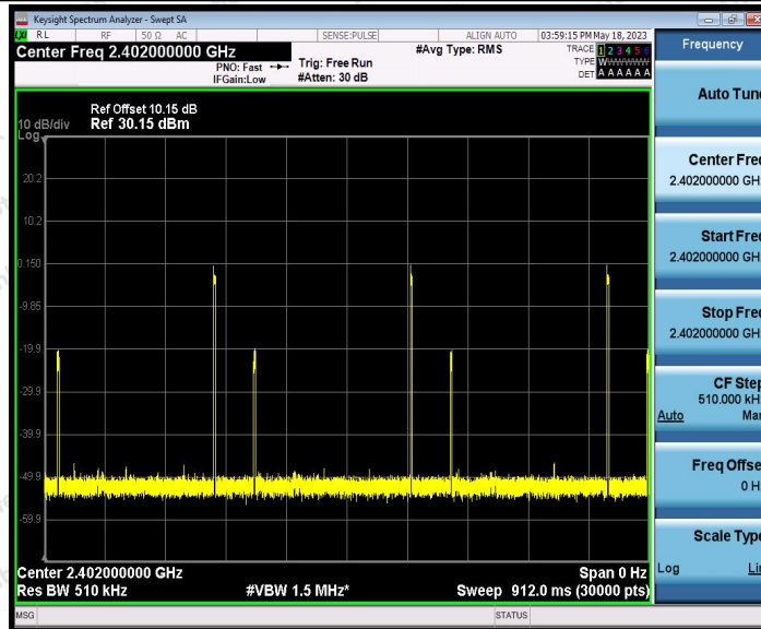
2DH5_Ant1_Hop_2480
