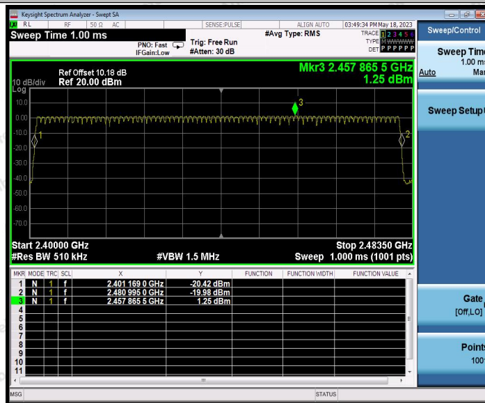
DH5_Ant1_Hop_2480
