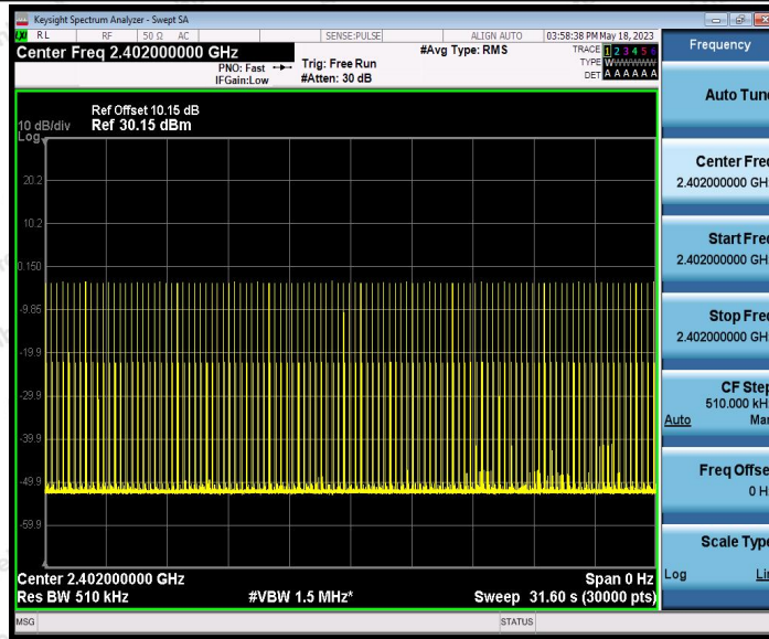
2DH5_Ant1_Hop_2480
