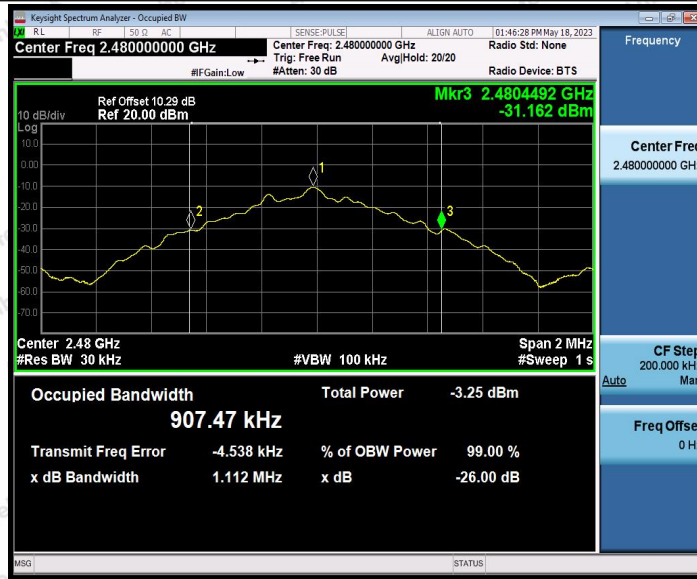
DH5_Ant1_2402
