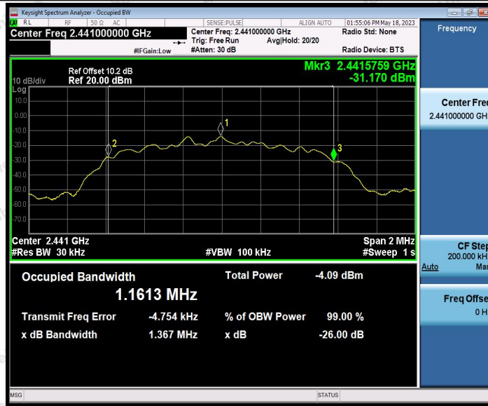
2D41_Ant1_2480
