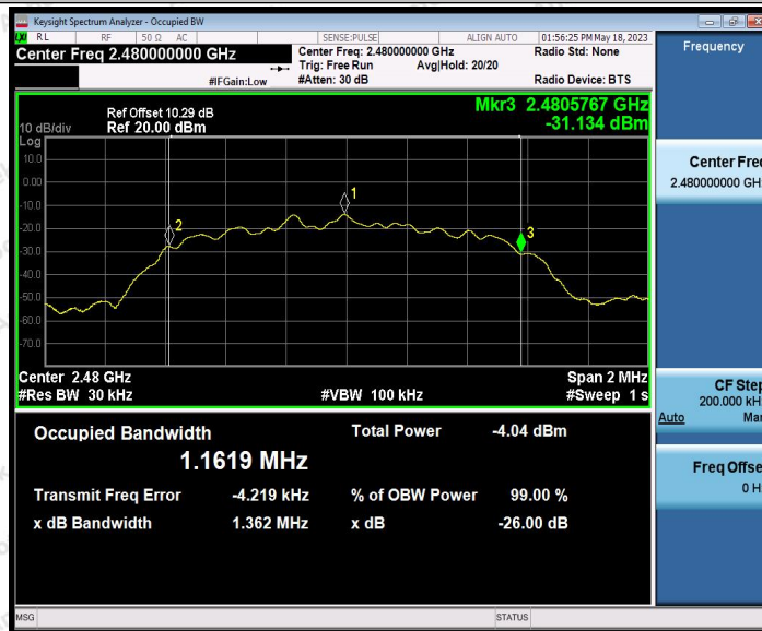
2D48_Ant1_2480
